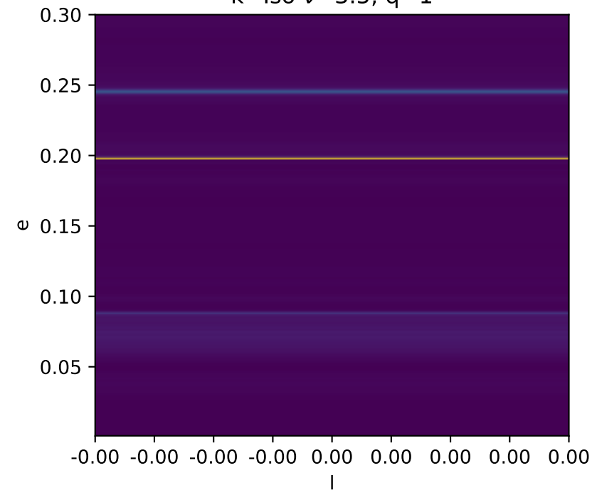
k=Iso \nu=3.5 , q=1
